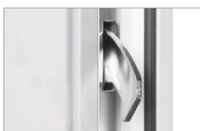
Рейкові замки BLUEMATIC EAV3 з протизламними ригелями. Рівень протизламності RC3.
