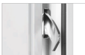
Рейкові замки BLUEMATIC EAV3 з протизламними ригелями. Рівень протизламності RC3.
